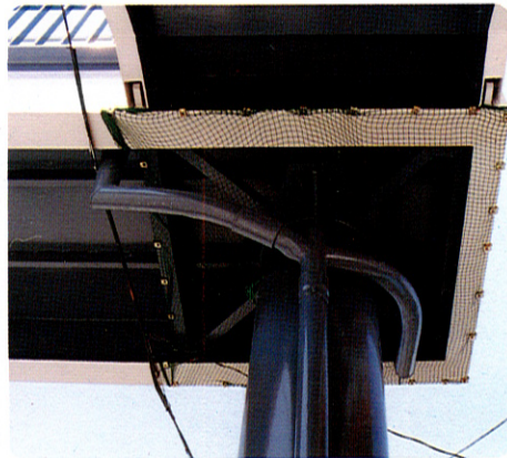
ネット/ポリエチレン・ナイロン 留め金具/パイラックス
