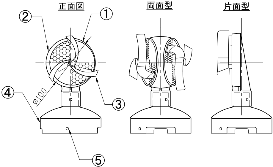
頭部詳細図
