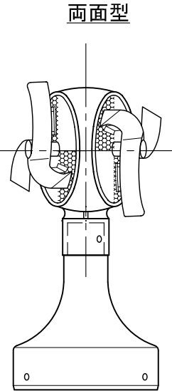
頭部詳細図
