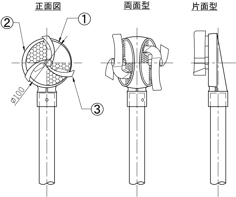
頭部詳細図
