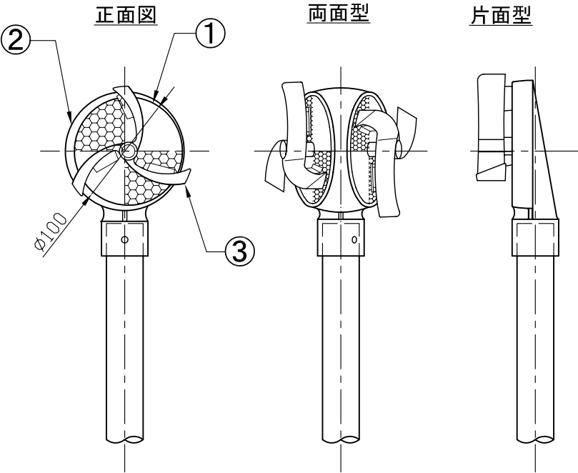
頭部詳細図
