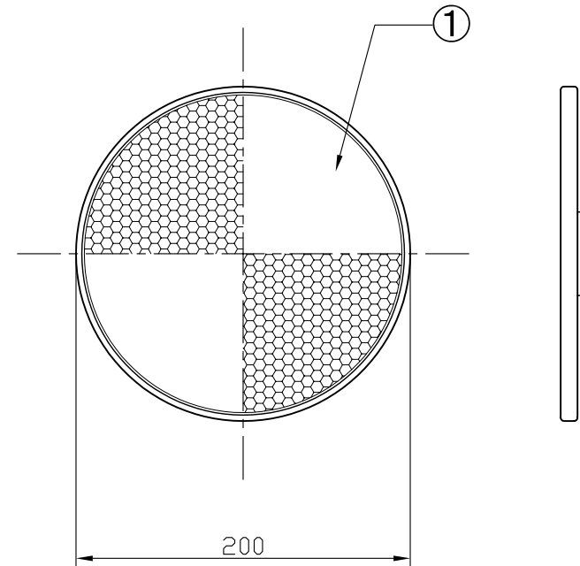
頭部詳細図
