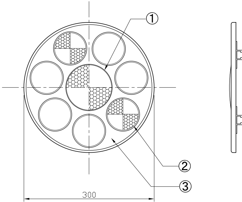
頭部詳細図
