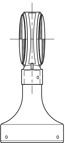
視線誘導標 CGR-100 (φ100両面・片面) ガードレールキャップ式
